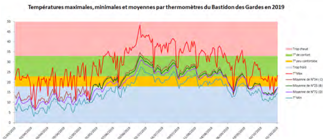
Figure 2 : Graphique des températures maximales, minimales et moyennes par thermomètres du Bastidon des Gardes en 2019.
